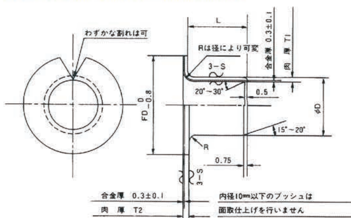
鋳付クリーンメタル標準品図面 Standard diagram for flanged Clean Metal bearings
